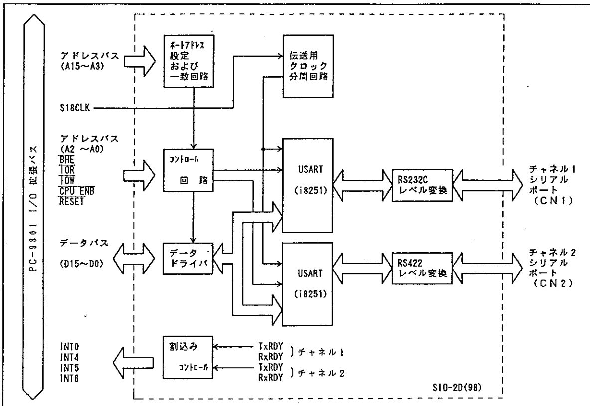
回路ブロック図
