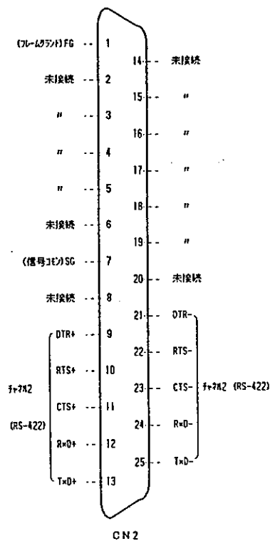
外部接続コネクタ信号配置
