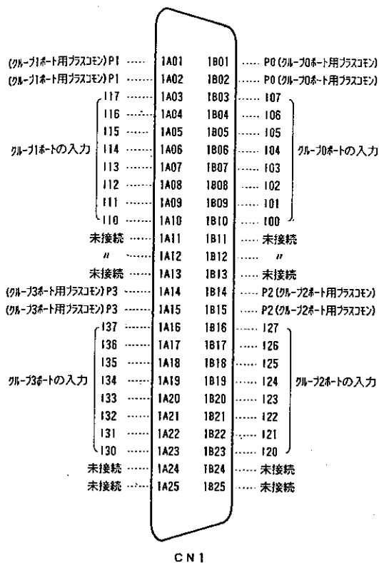
外部接続コネクタ信号配置
