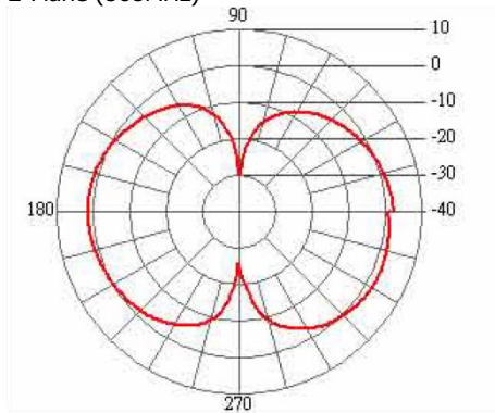
E-Plane (868MHz)
