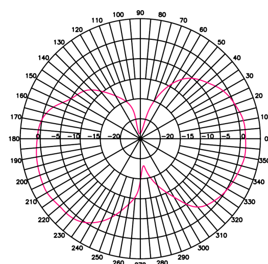
E-Plane (925MHz)
