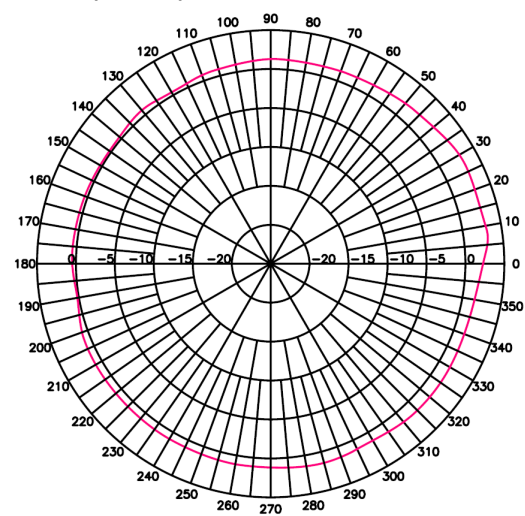
AI-1004LY-WQ-US H-Plane (925MHz)
