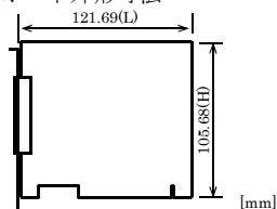
ボード外形寸法
