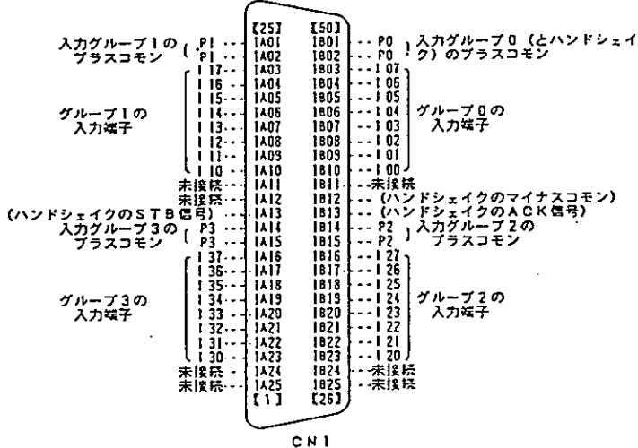
外部接続コネクタ信号配置
